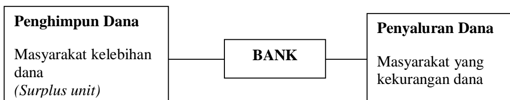
Gambar 2.1. Bagan Bank Lembaga Perantara Keuangan
