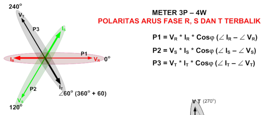
Gambar 2.14 Polaritas Terbalik
