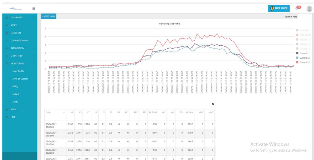
Gambar 4.13 Tampilan Profile Energi Per Pelanggan
