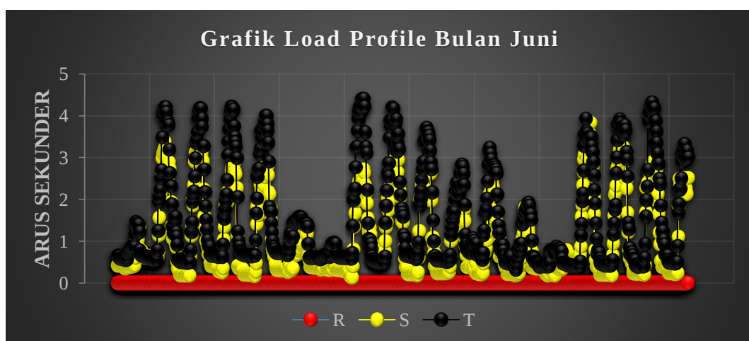
Gambar 4.3 Grafik Load Profile Bulan Juni
