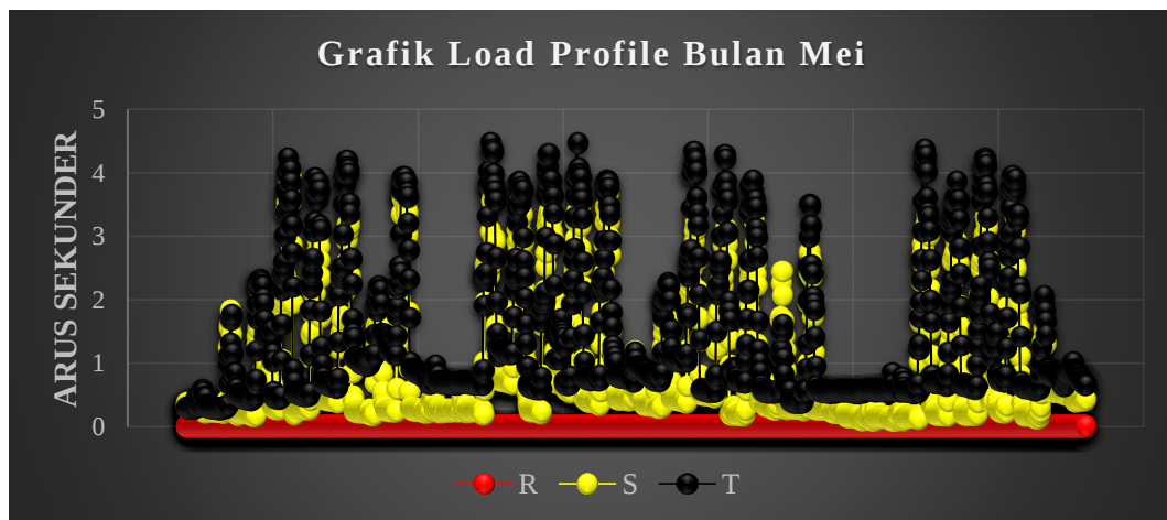
Gambar 4.2 Grafik Load Profile Bulan Mei
