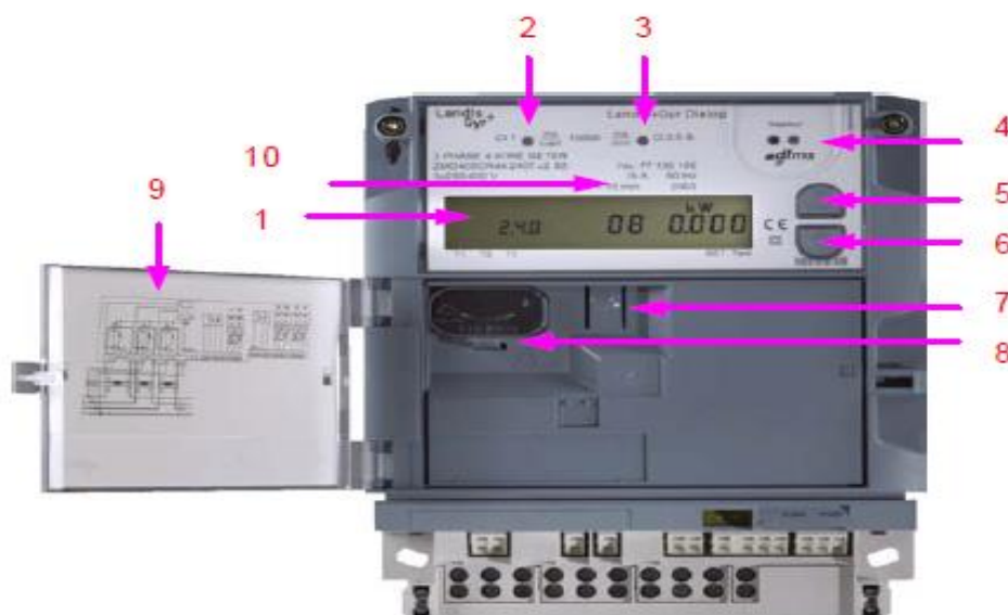
Gambar 2.4 Display meter
