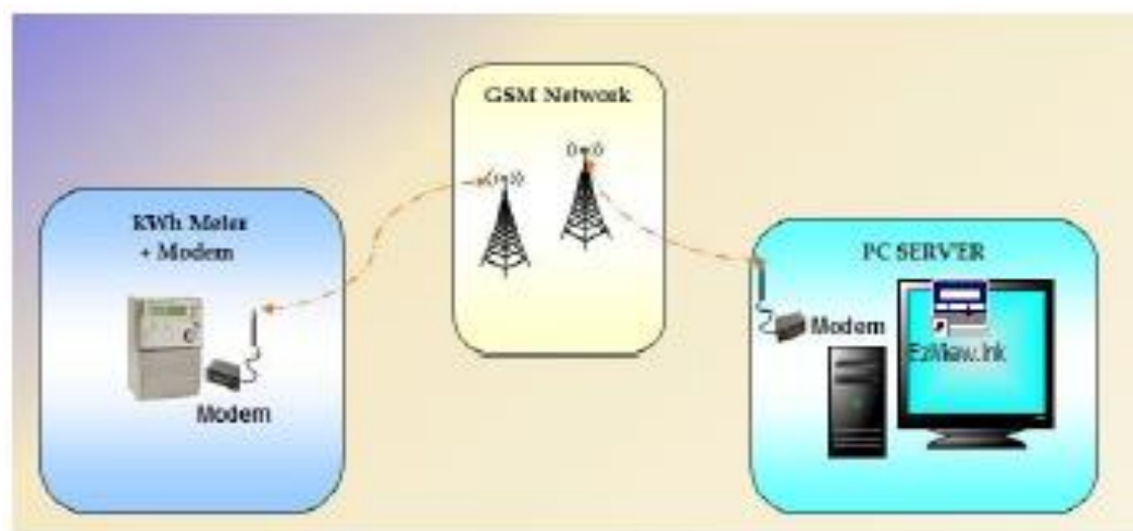
Gambar 4.11 Proses Pembacaan Meter
