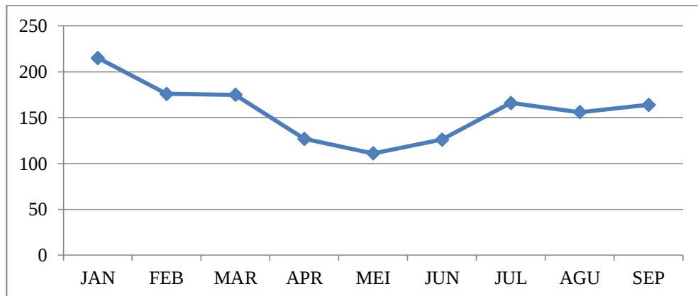
Gambar 4.5 Grafik Jam Nyala Pelanggan
