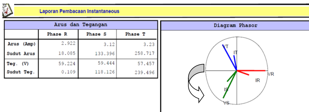
Gambar 2.11 Phasor Beban Induktif
