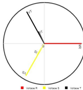
Gambar 4.6 Diagram phasor yang mengalami anomaly / kejanggalan
