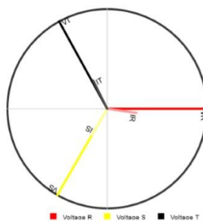
Gambar 4.7 Diagram phasor yang benar/sesuai
