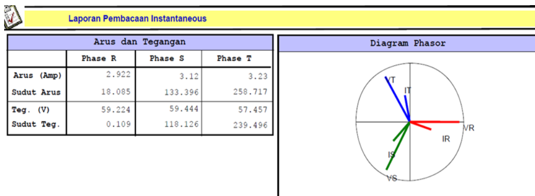
Gambar 2.10 Phasor Kondisi Normal
