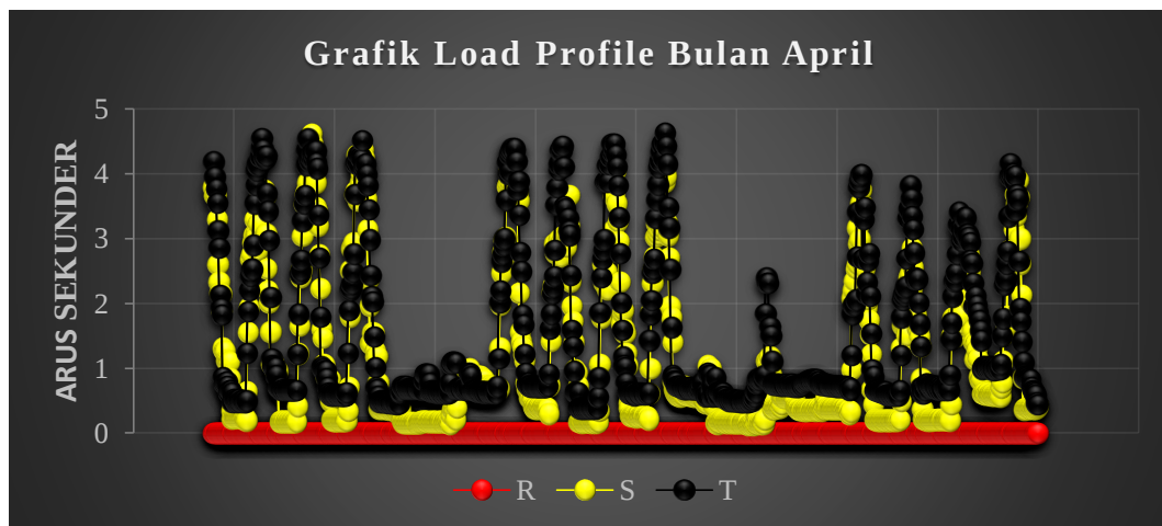
Gambar 4.1 Grafik Load Profile Bulan April
